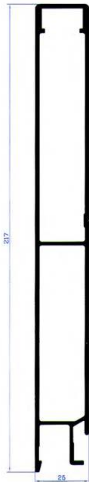
PA-201 Προφίλ κεφαλάρι Βάρος 2670 gr/m
