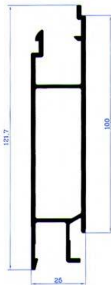
PA-205 Προφίλ μικρής σκάφης Βάρος 2506 gr/m
