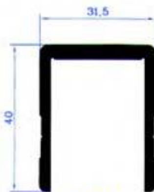
PA-211 Προφίλ Πι παραπετών Βάρος 880 gr/m
