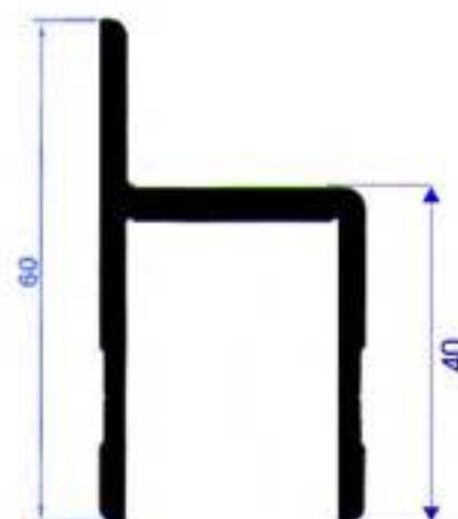
PA-212 Προφίλ Πι με φτερό Βάρος 1040 gr/m
